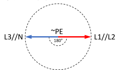
Fig. 7) 1Φ3W / split phase
